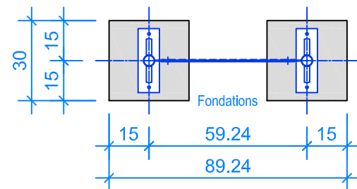
PLAN 1:20 PANNEAU D'INFORMATION
