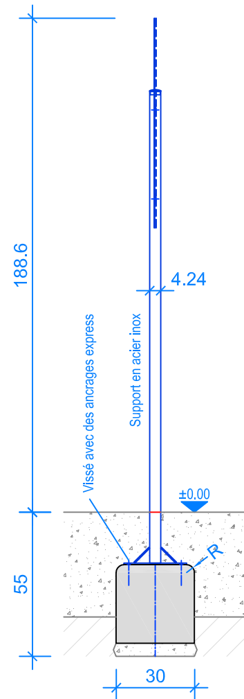
COUPE 1:20 PANNEAU D'INFORMATION
