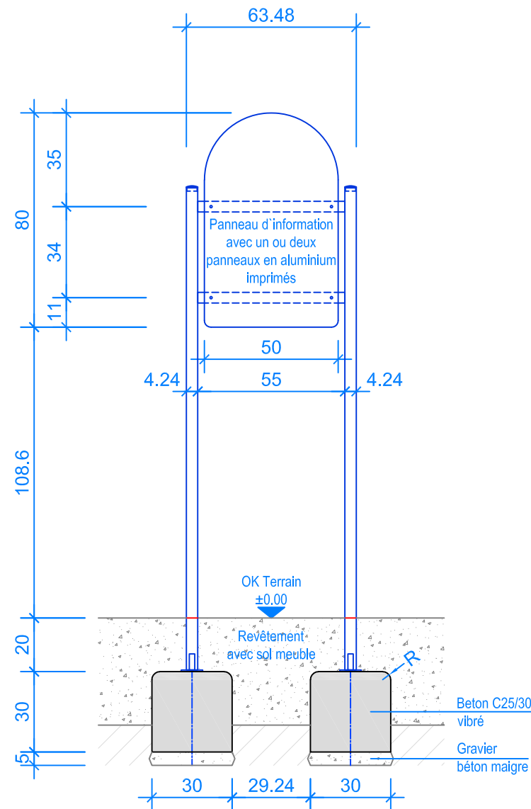
VUE 1:20 PANNEAU D'INFORMATION
