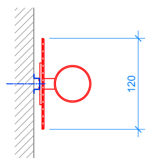
PLAN 1:50
