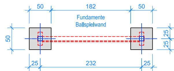
GRUNDRISS 1:50
