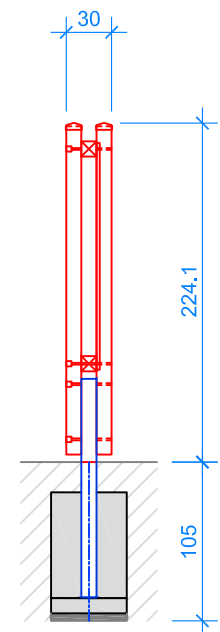
SCHNITT 1:50
