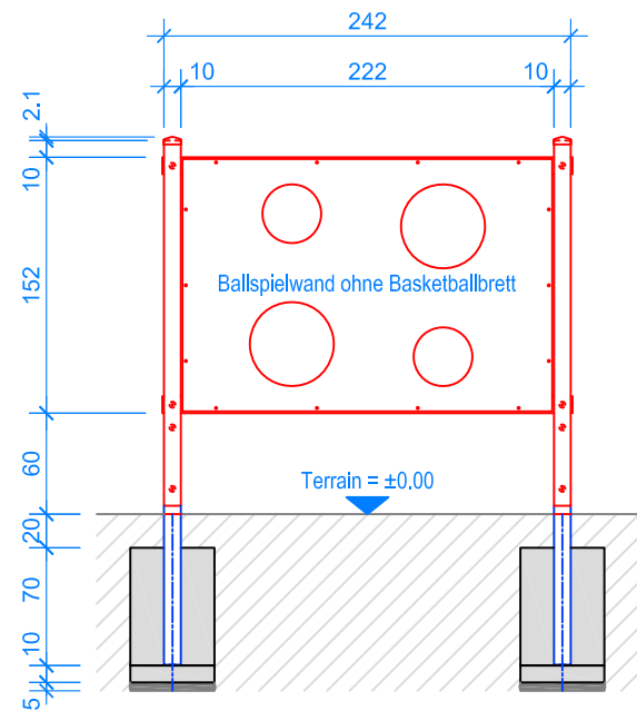
ANSICHT 1:50
