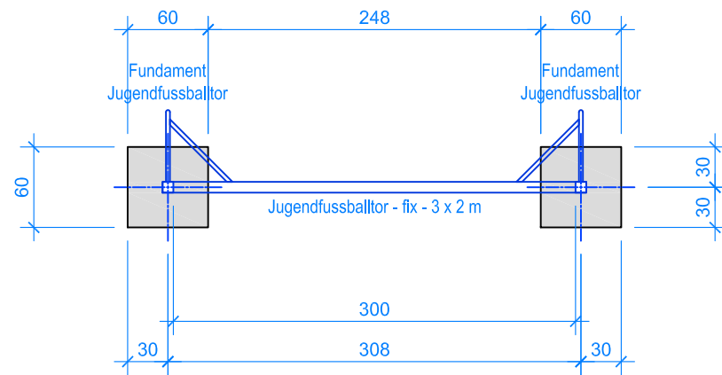
GRUNDRISS 1:50
