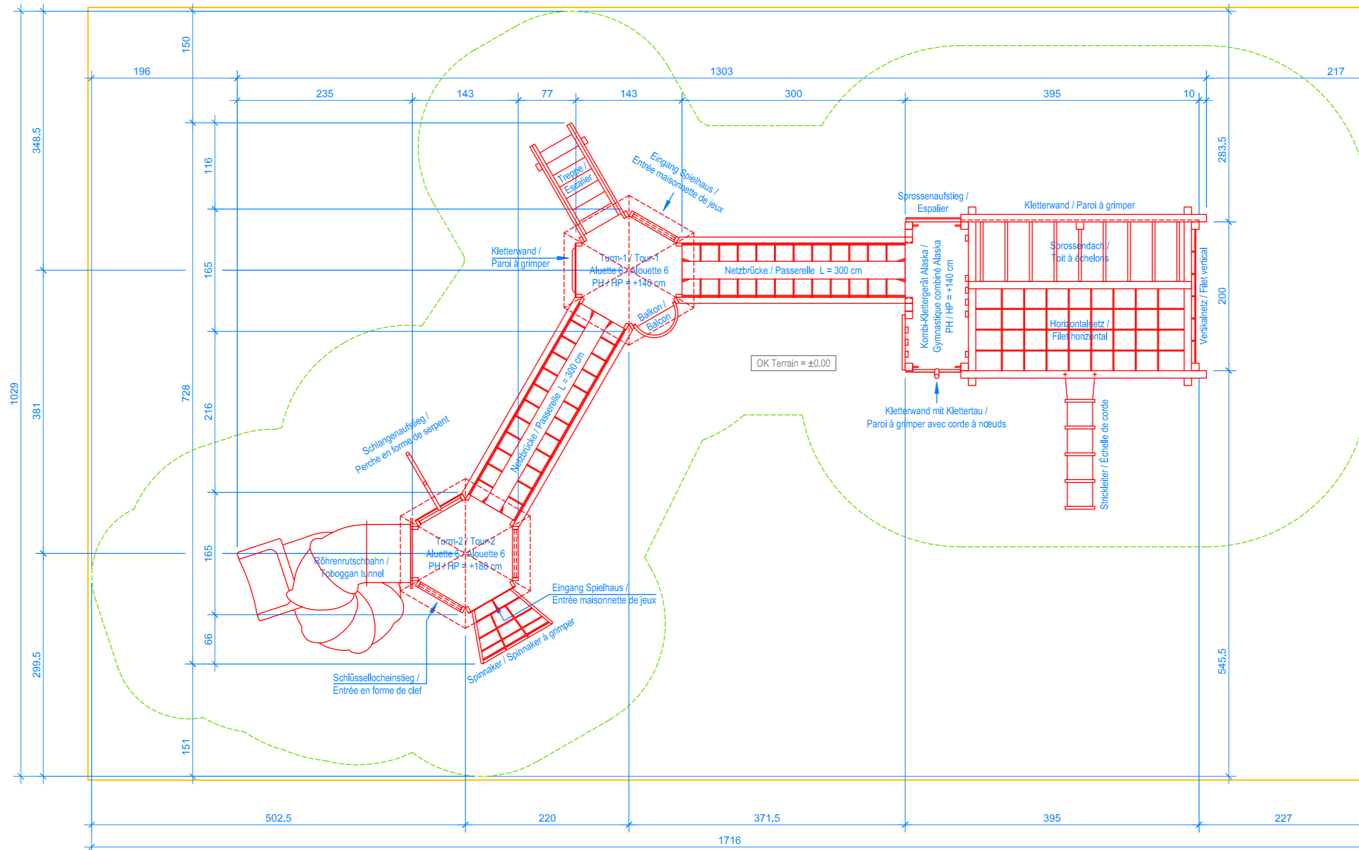
GRUNDRISS / PLAN 1:50
