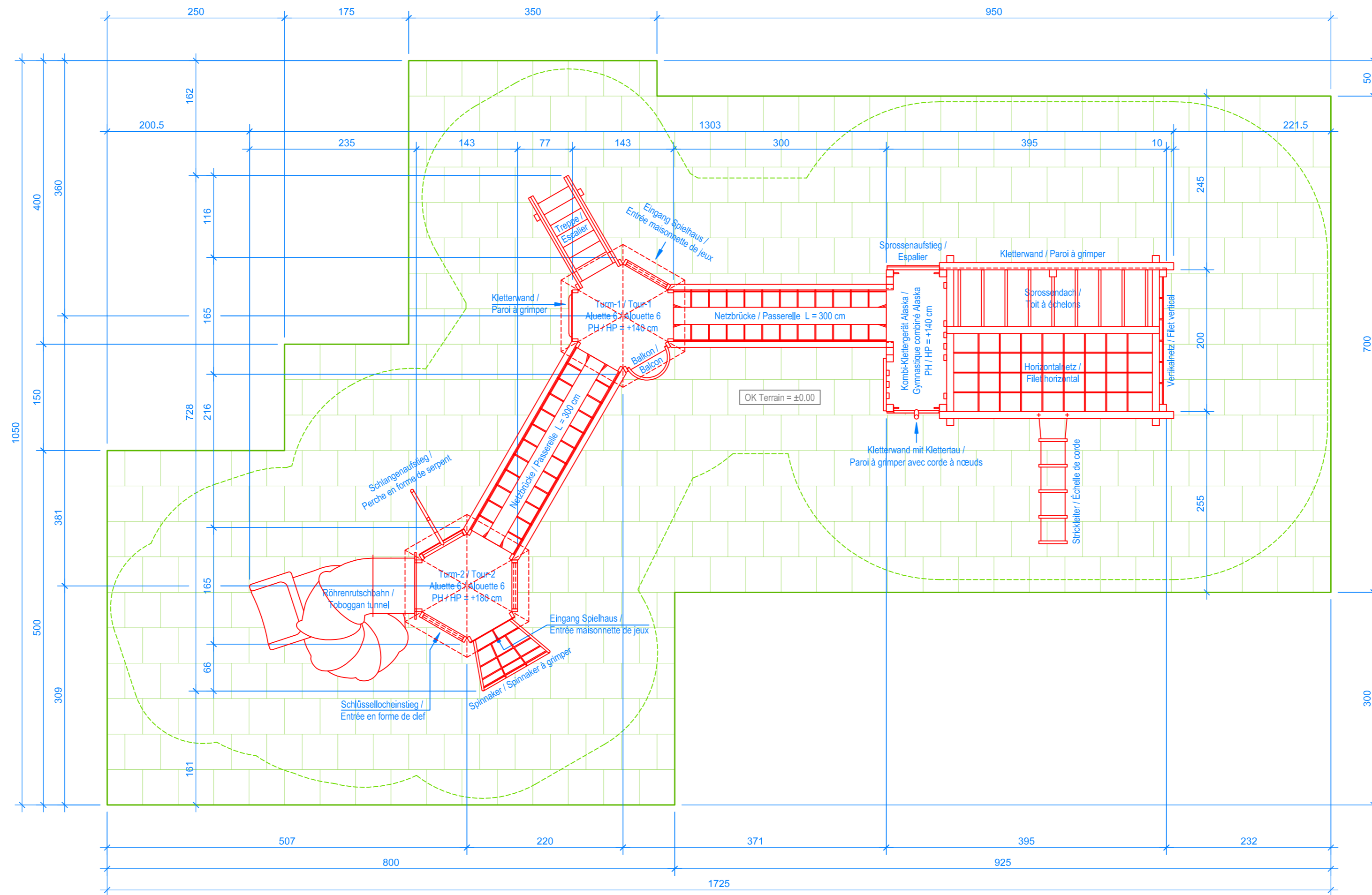
GRUNDRISS / PLAN 1:50
