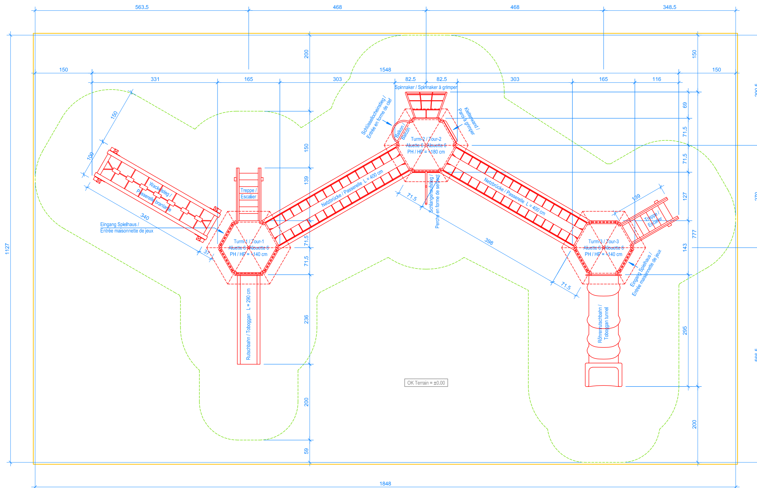
GRUNDRISS / PLAN 1:50
