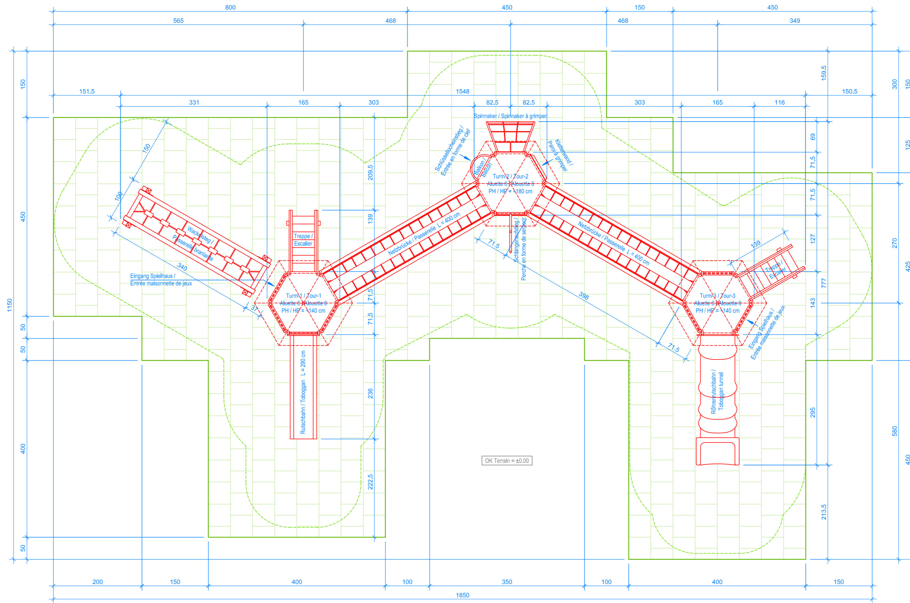
GRUNDRISS / PLAN 1:50
