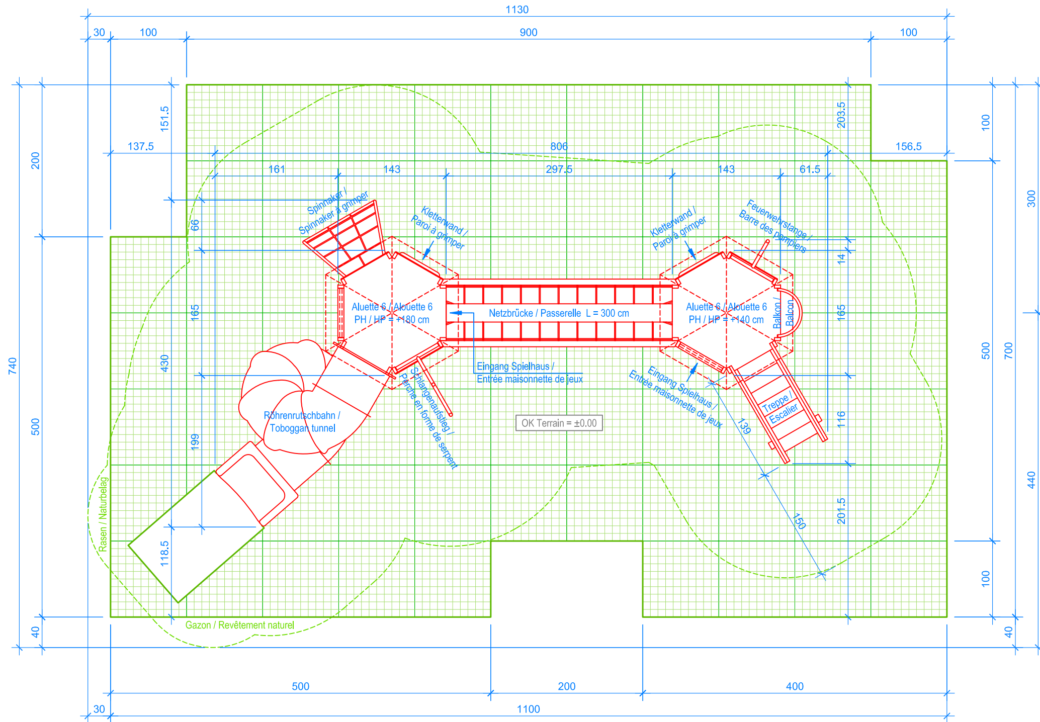
GRUNDRISS / PLAN 1:50
