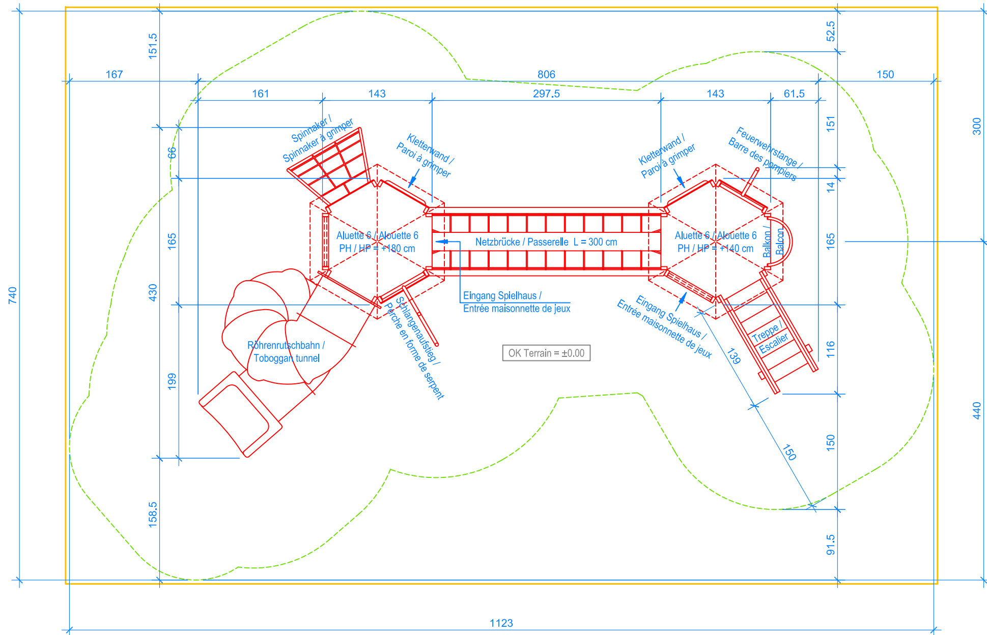
GRUNDRISS / PLAN 1:50
