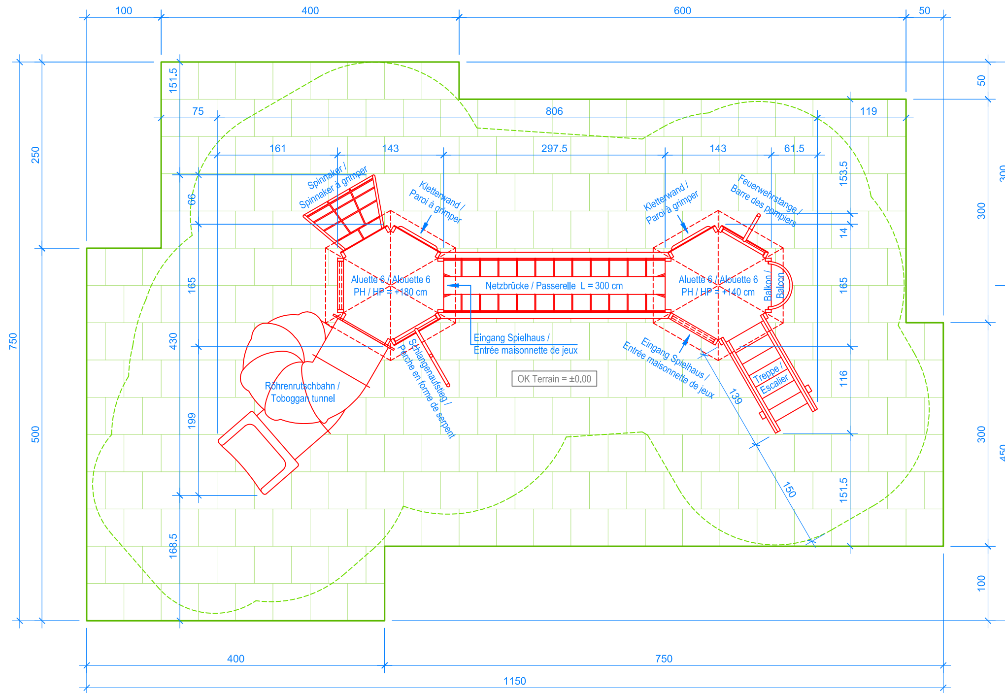
GRUNDRISS / PLAN 1:50
