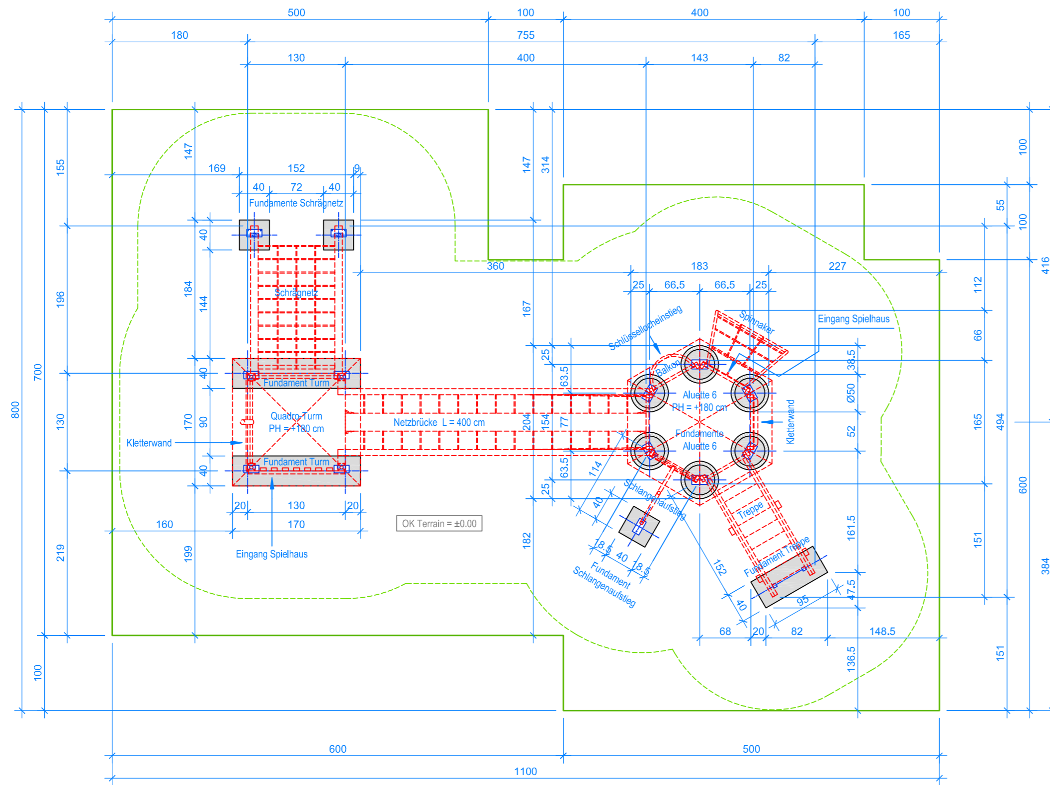
GRUNDRISS 1:50
