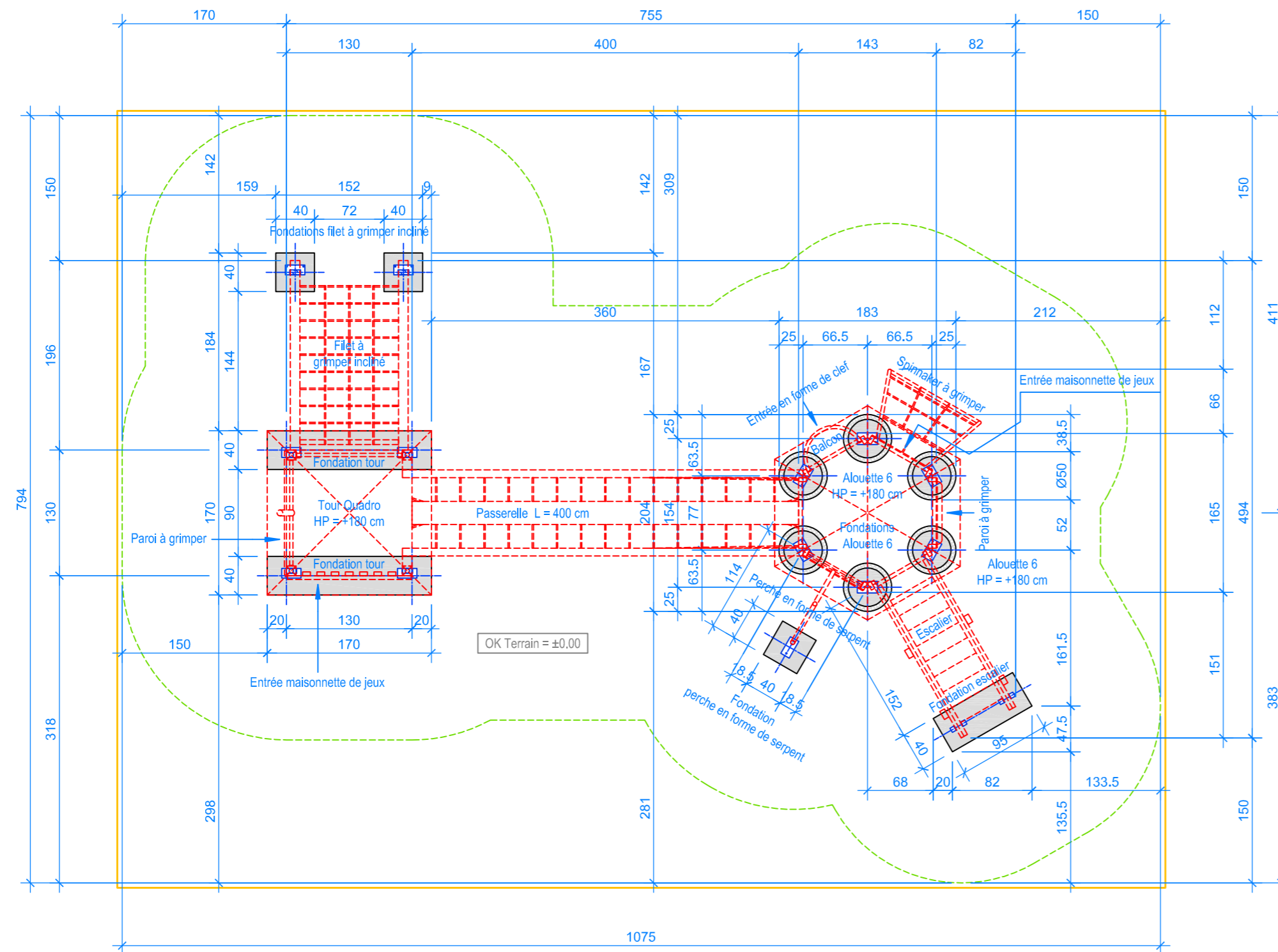
PLAN 1:50
