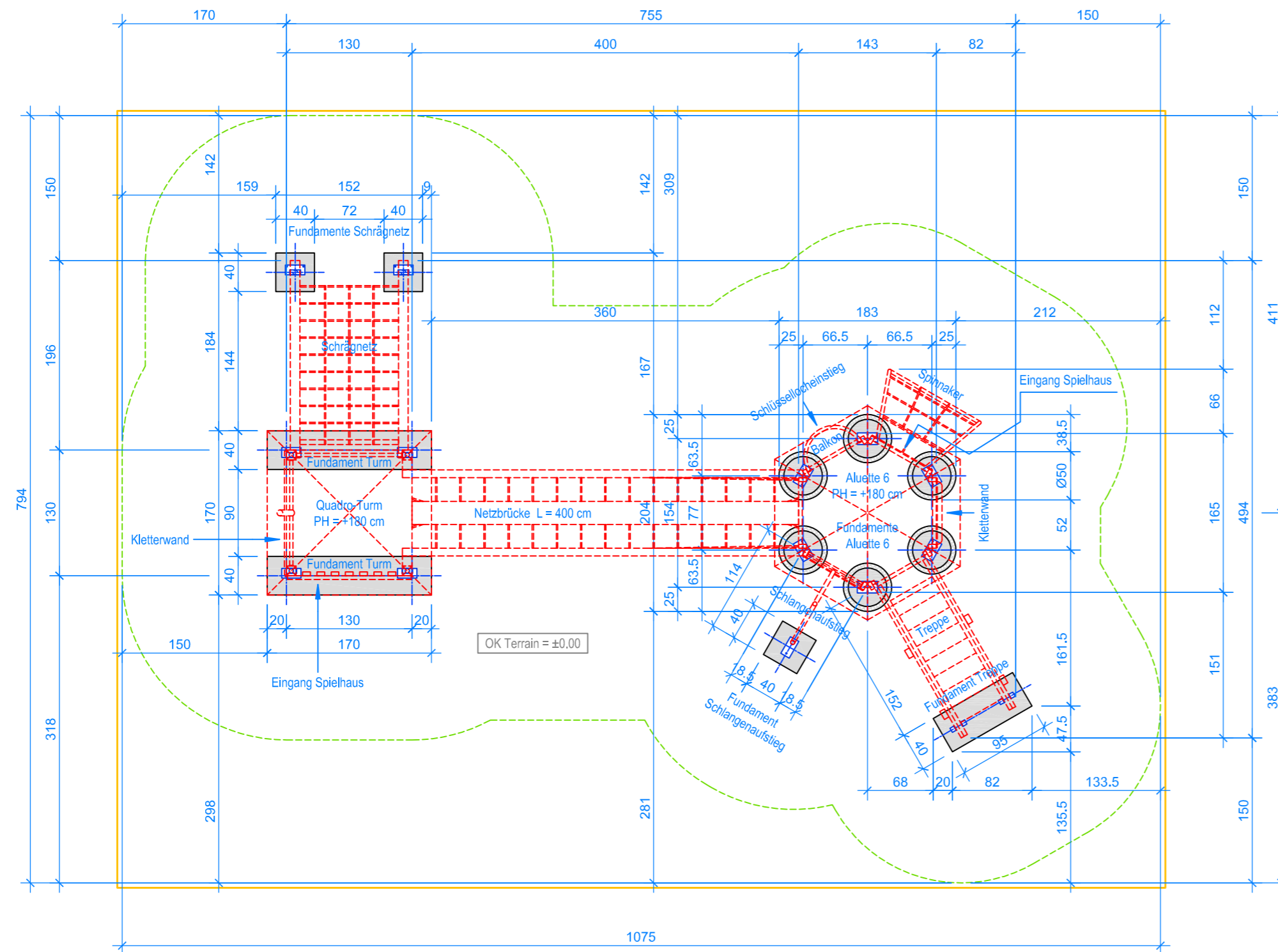
GRUNDRISS 1:50
