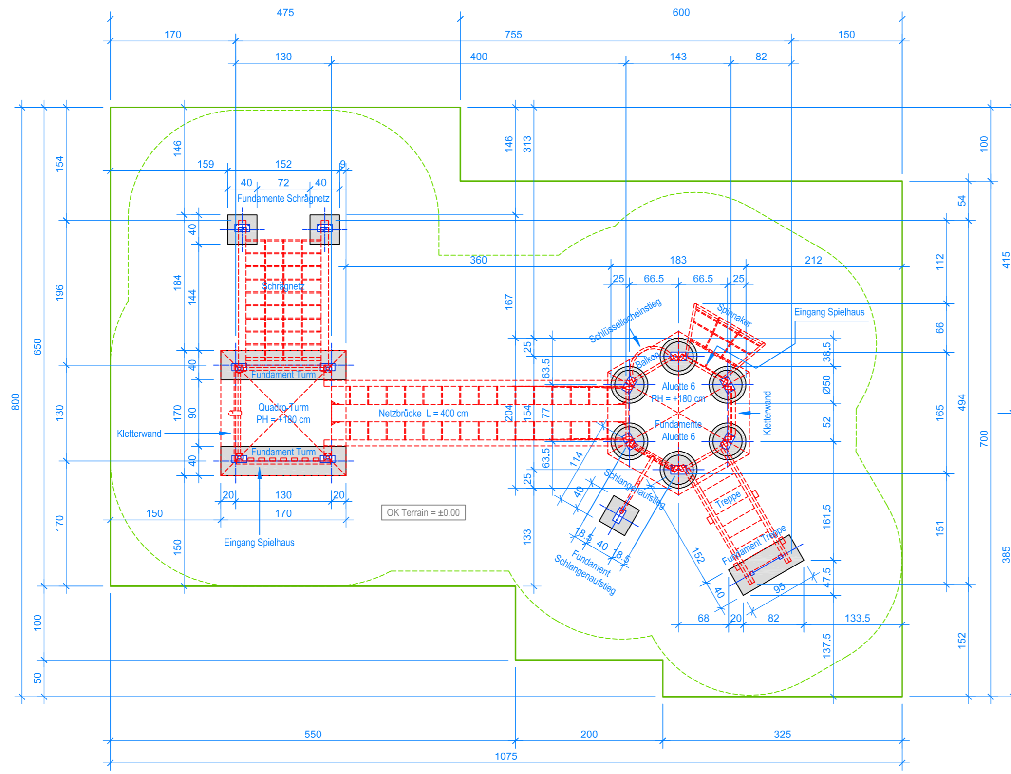
GRUNDRISS 1:50
