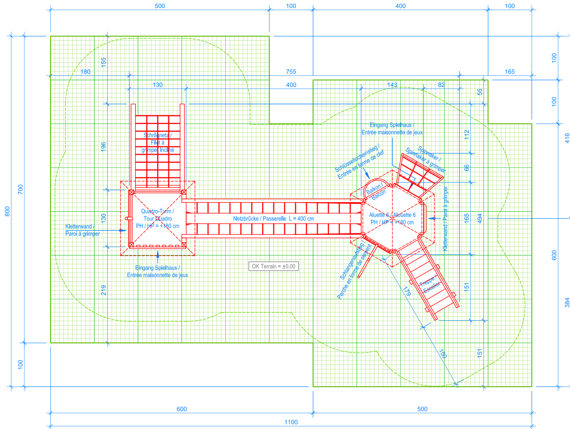
GRUNDRISS / PLAN 1:50
