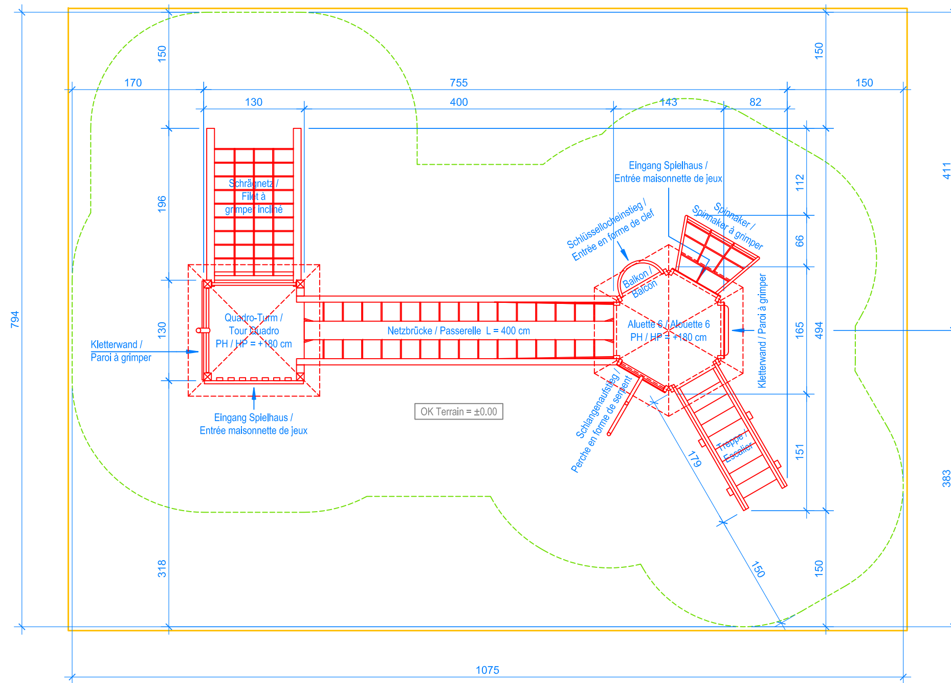
GRUNDRISS / PLAN 1:50
