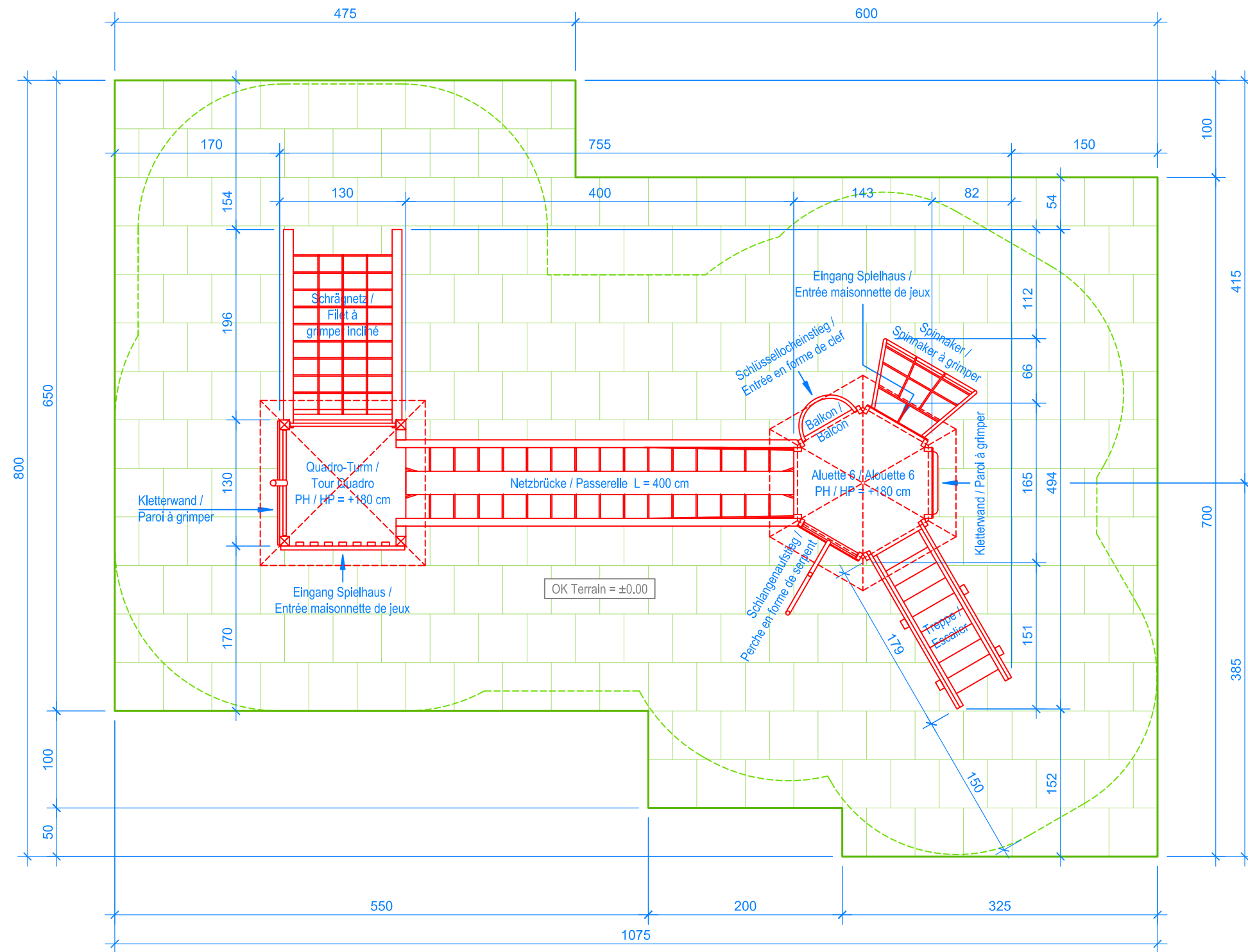
GRUNDRISS / PLAN 1:50
