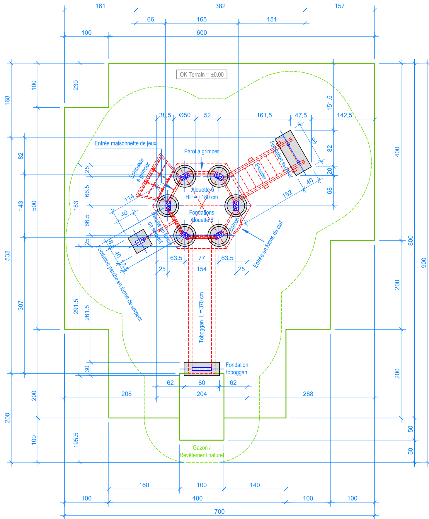
PLAN 1:50
