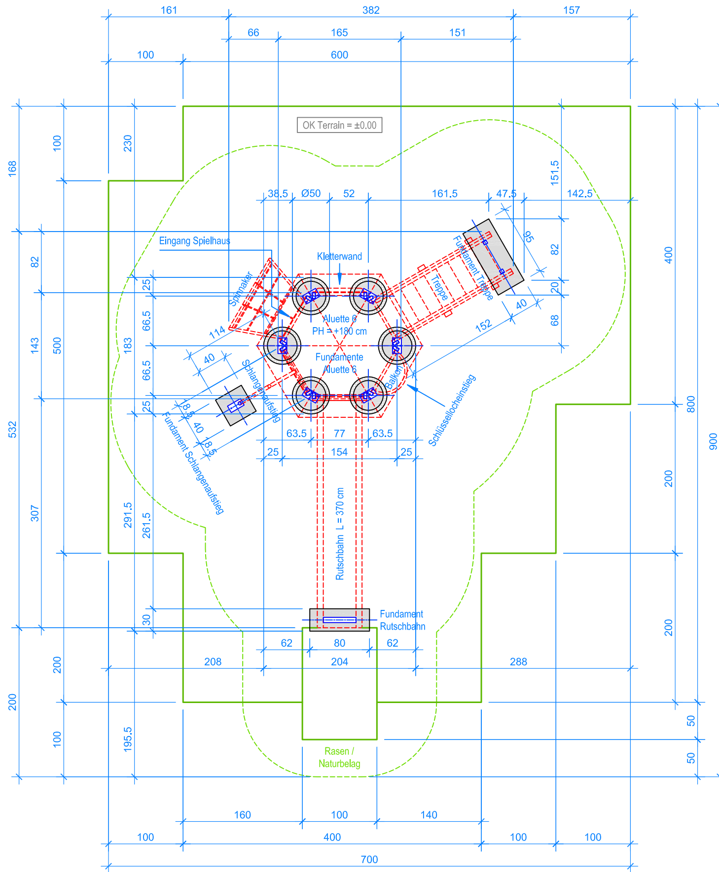
GRUNDRISS 1:50
