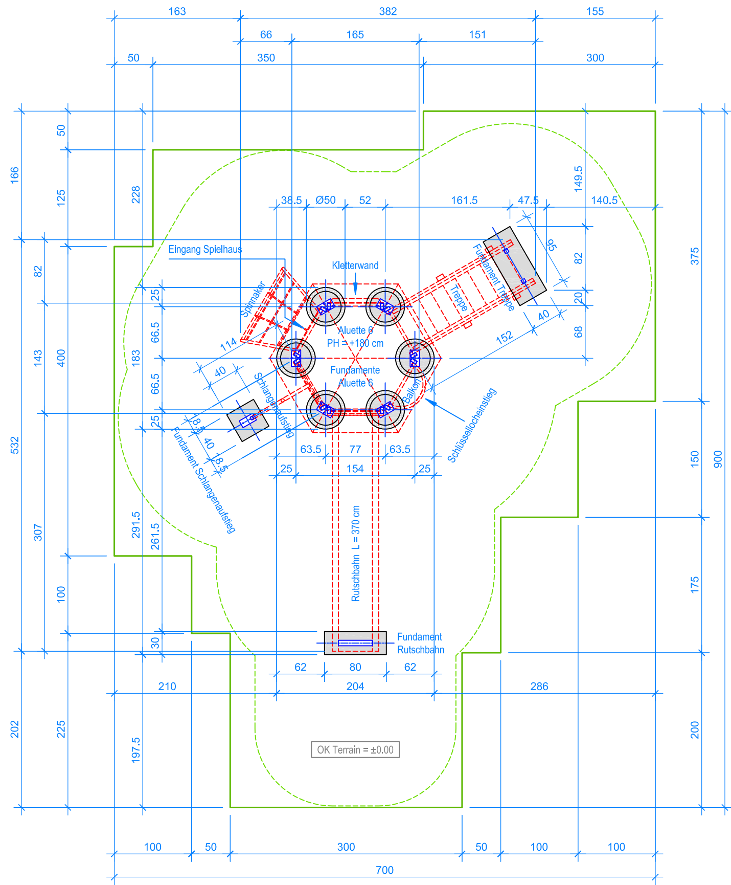
GRUNDRISS 1:50
