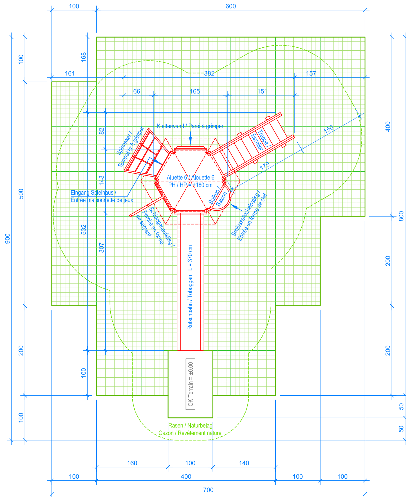
GRUNDRISS / PLAN 1:50
