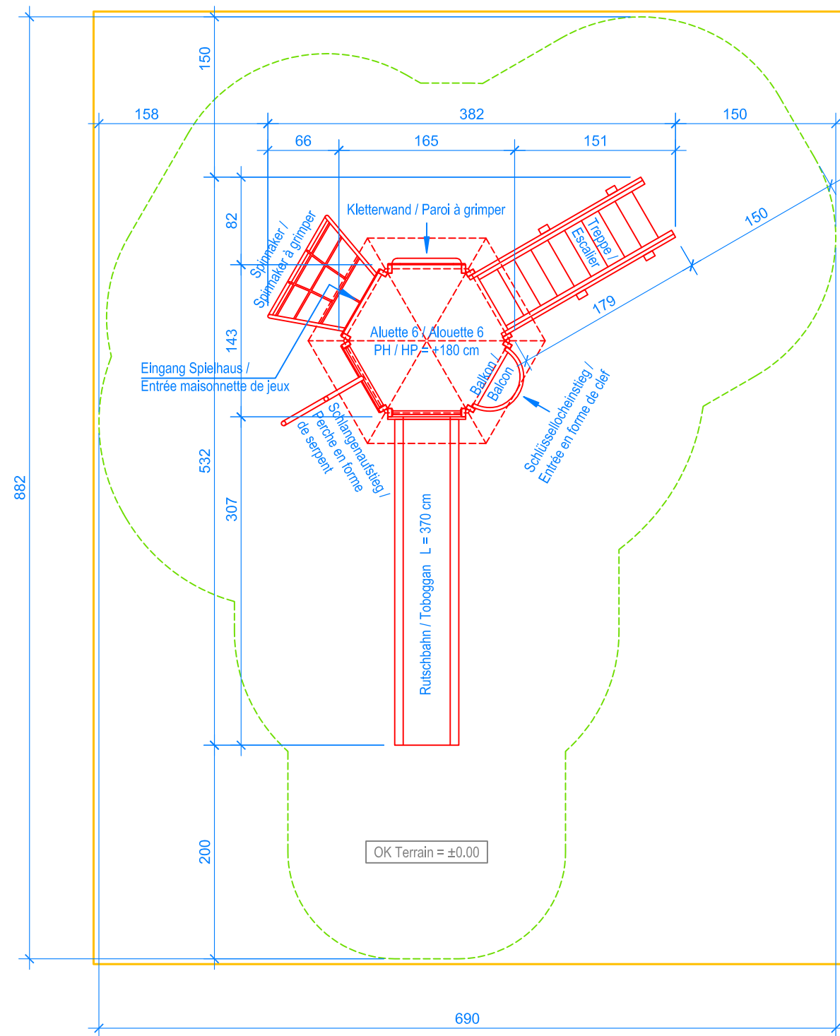
GRUNDRISS / PLAN 1:50
