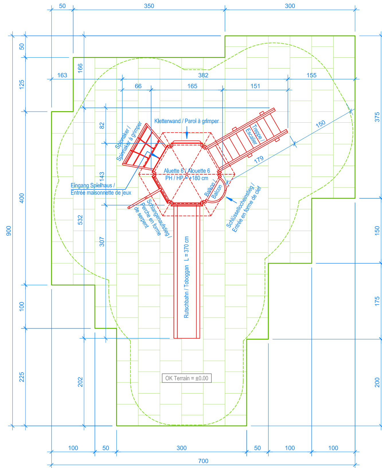
GRUNDRISS / PLAN 1:50
