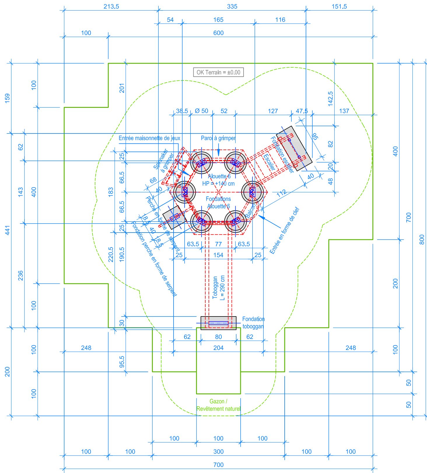
PLAN 1:50
