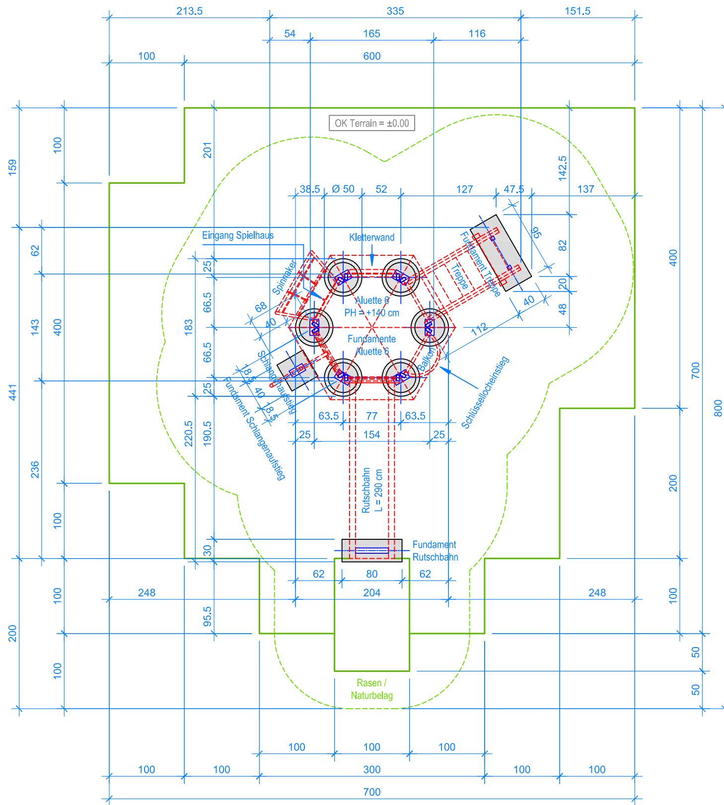
GRUNDRISS 1:50
