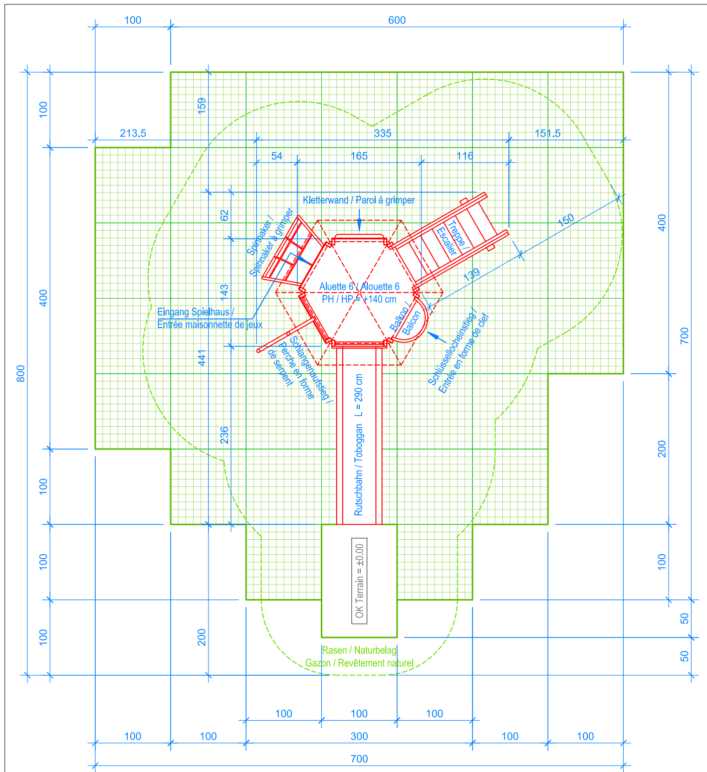
GRUNDRISS / PLAN 1:50
