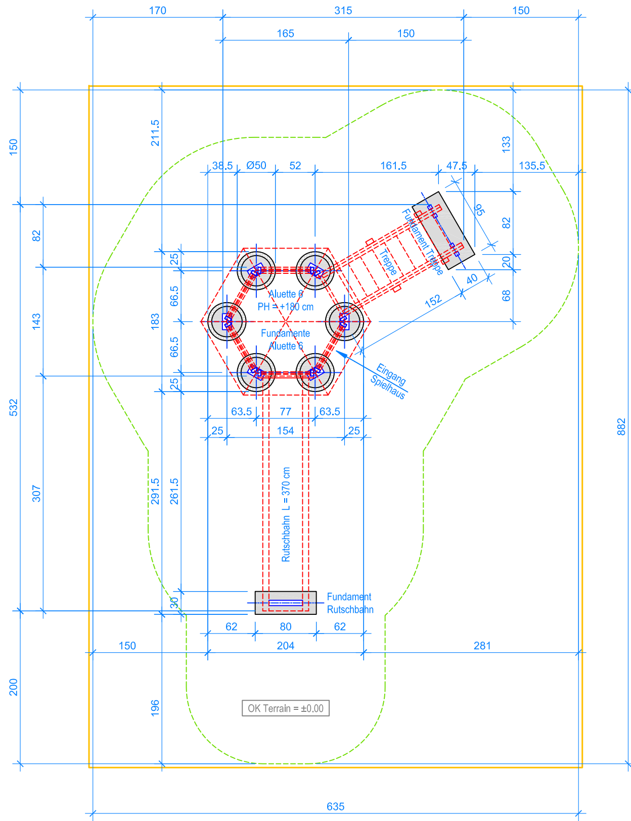
GRUNDRISS 1:50
