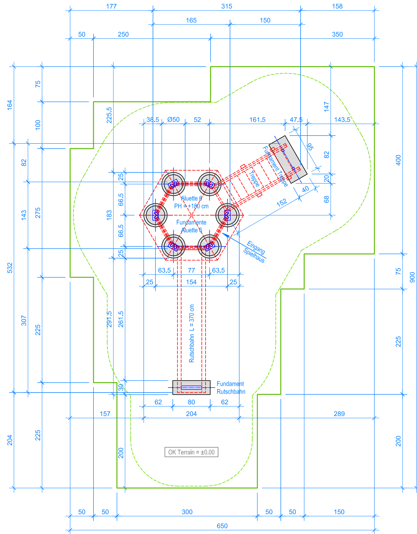
GRUNDRISS 1:50
