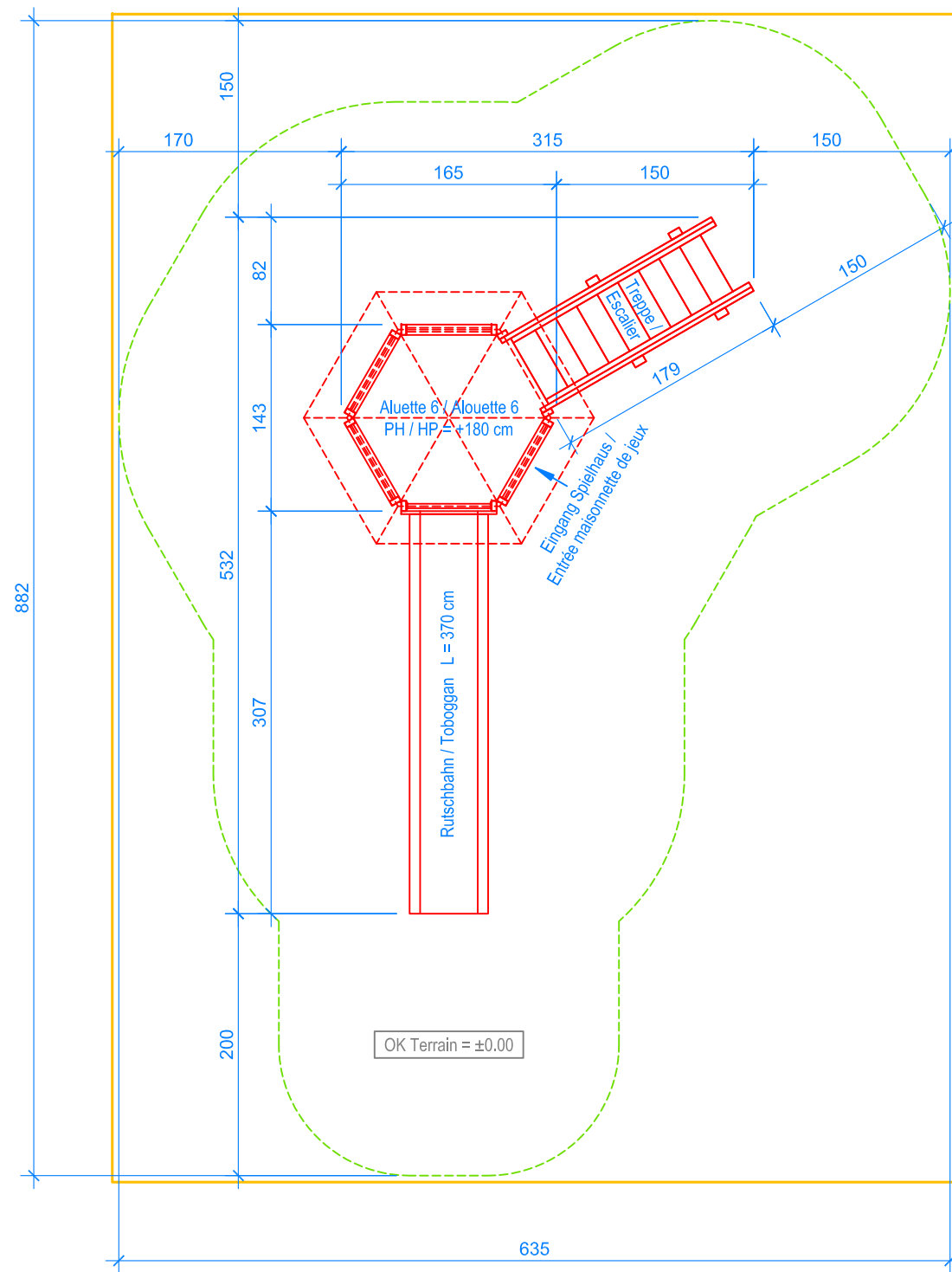
GRUNDRISS / PLAN 1:50
