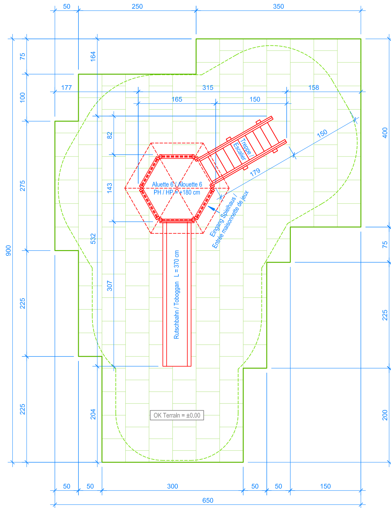
GRUNDRISS / PLAN 1:50
