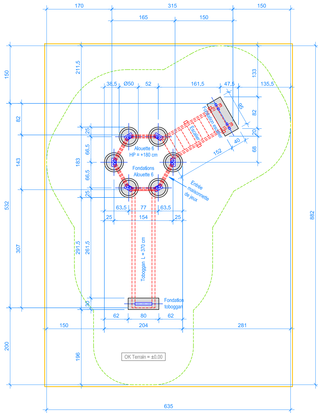
PLAN 1:50
