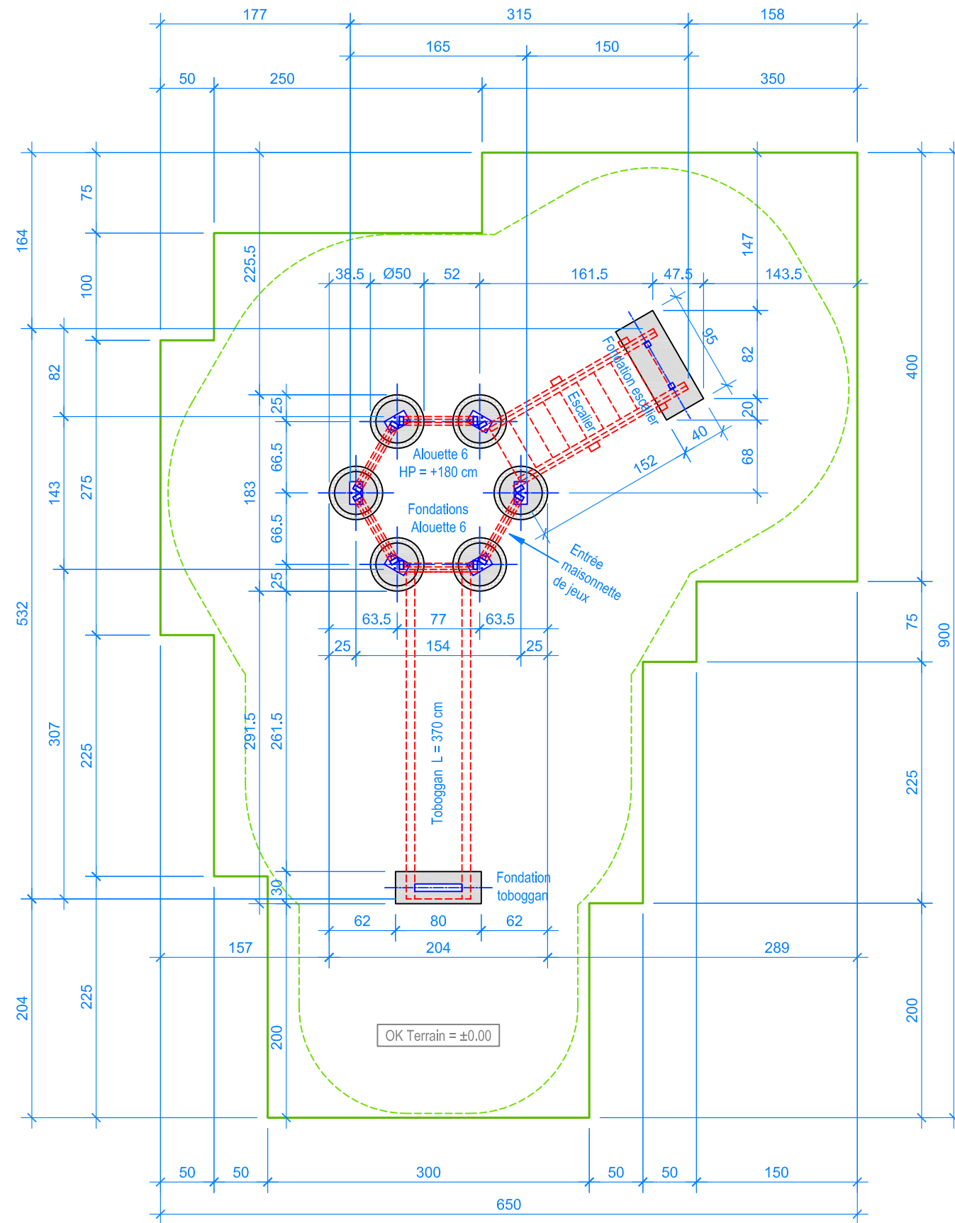
PLAN 1:50
