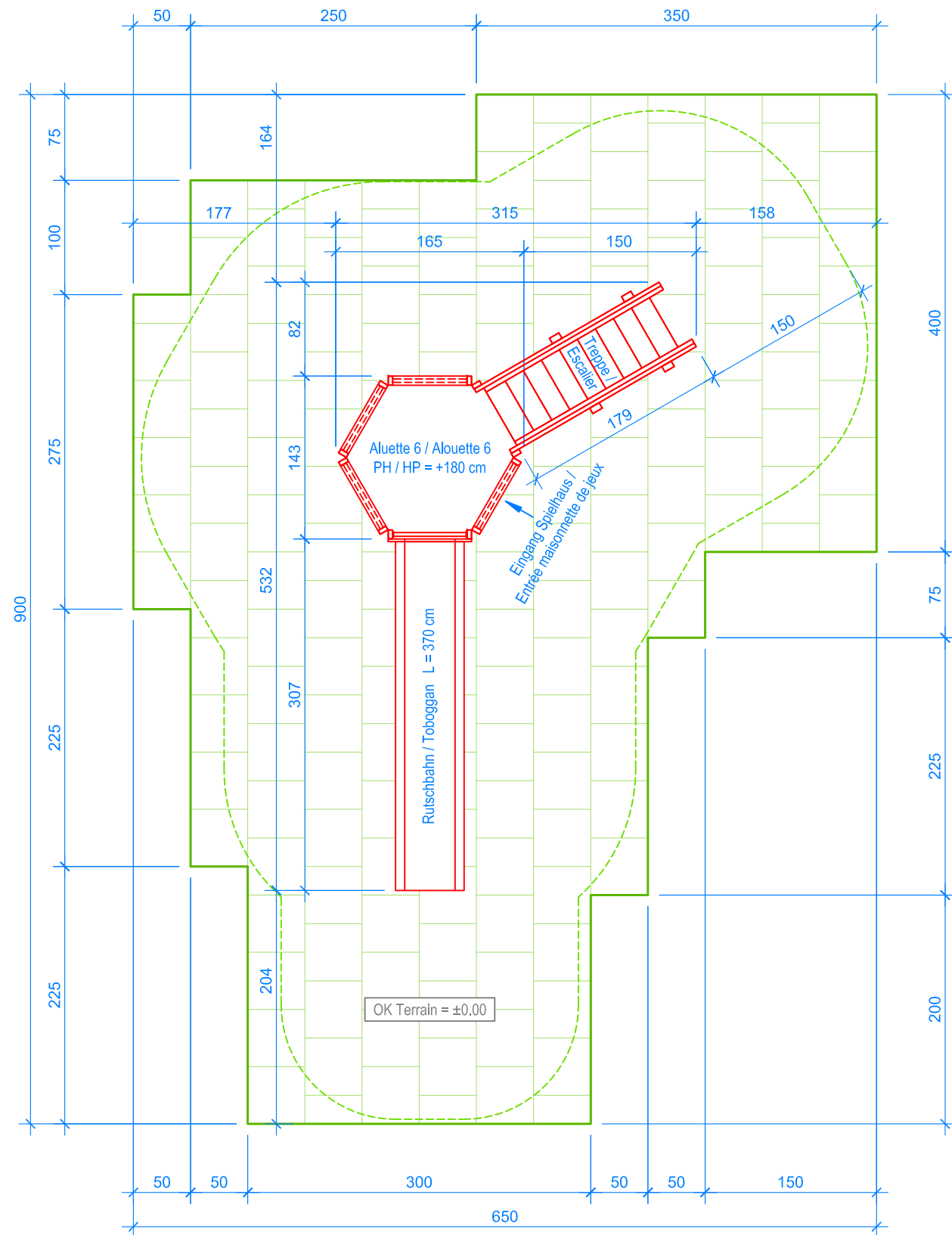
GRUNDRISS / PLAN 1:50
