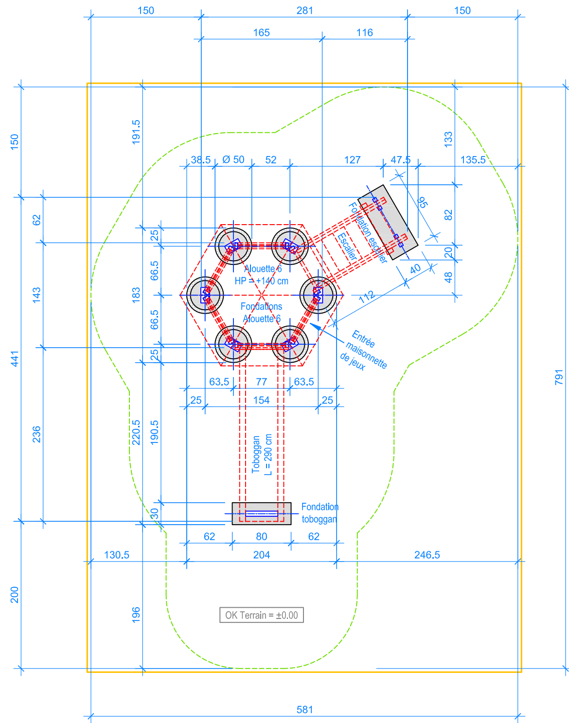
PLAN 1:50
