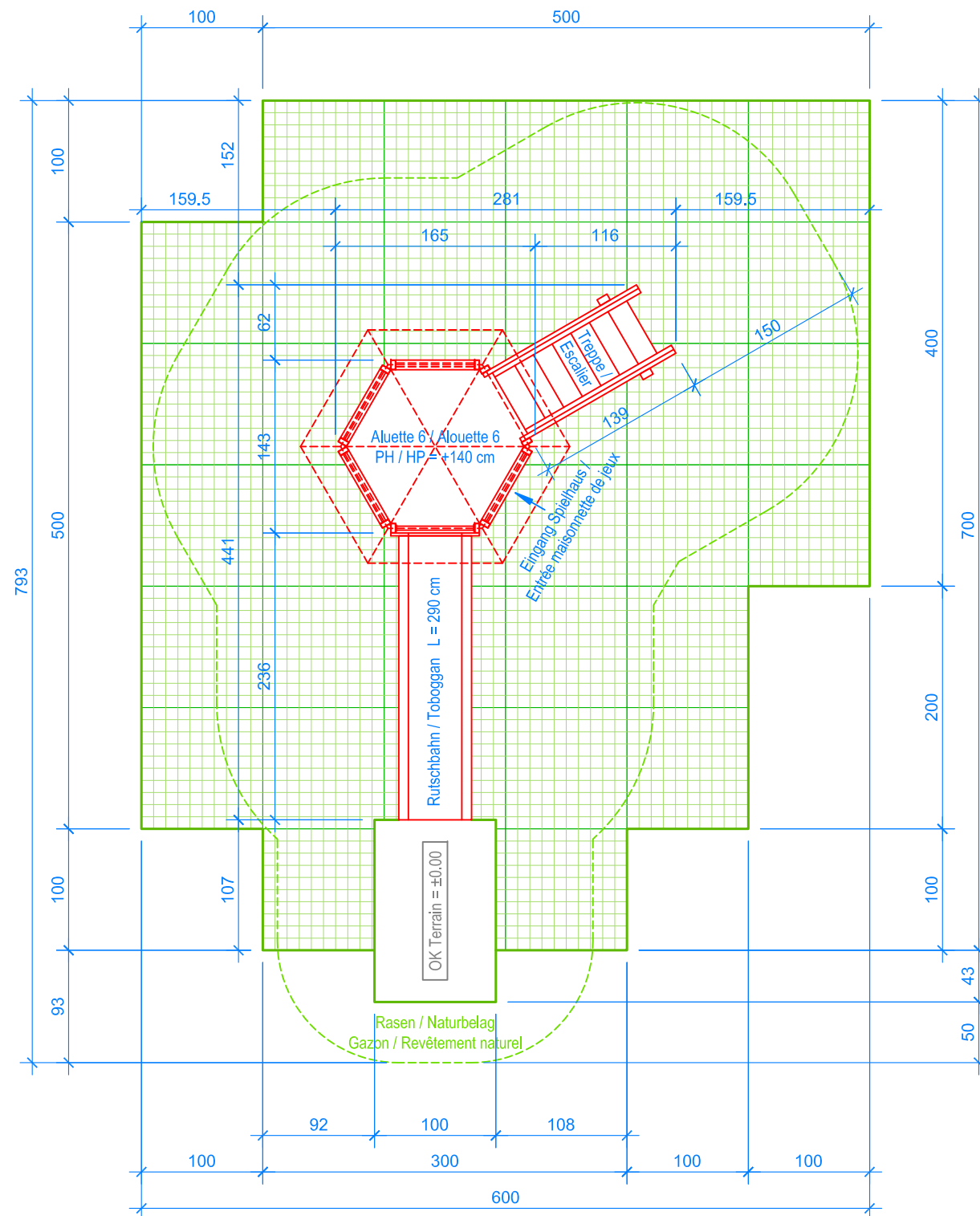
GRUNDRISS / PLAN 1:50
