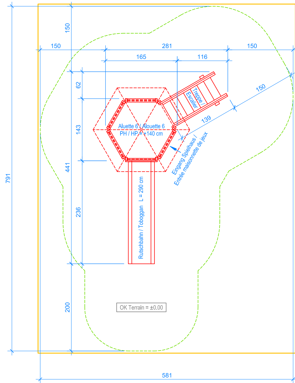
GRUNDRISS / PLAN 1:50
