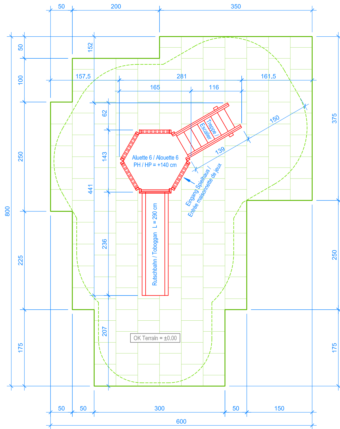
GRUNDRISS / PLAN 1:50
