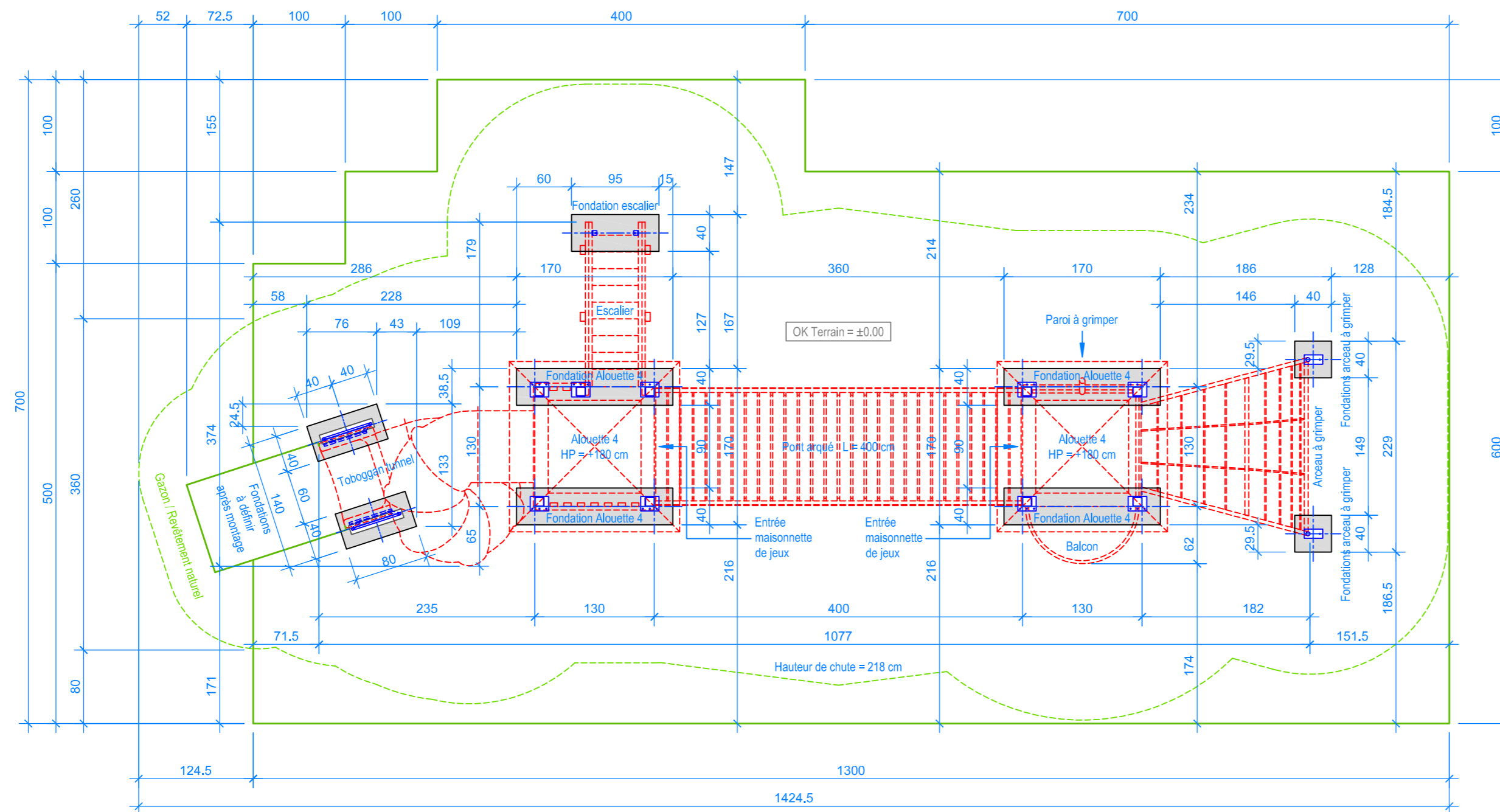
PLAN 1:50
