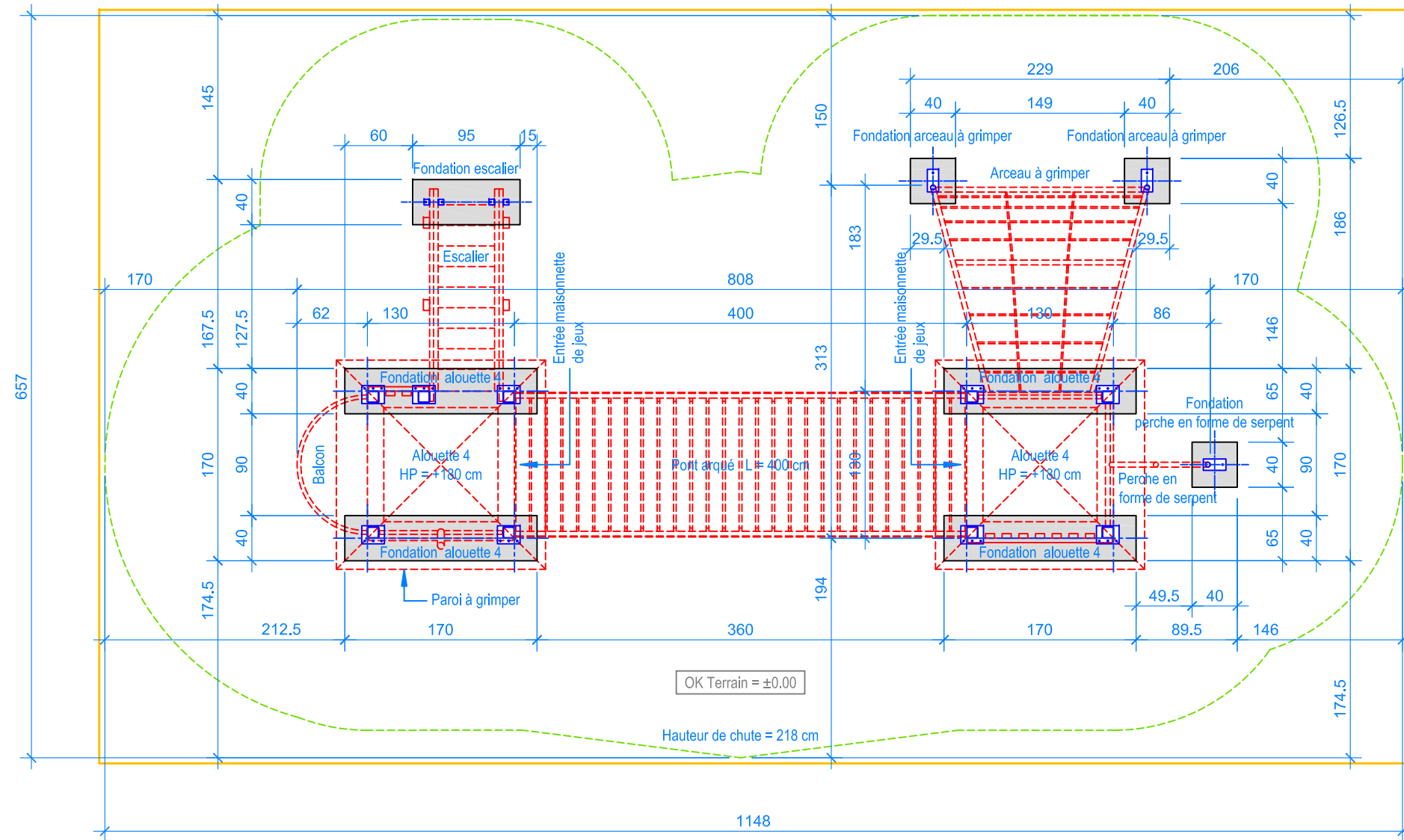
PLAN 1:50
