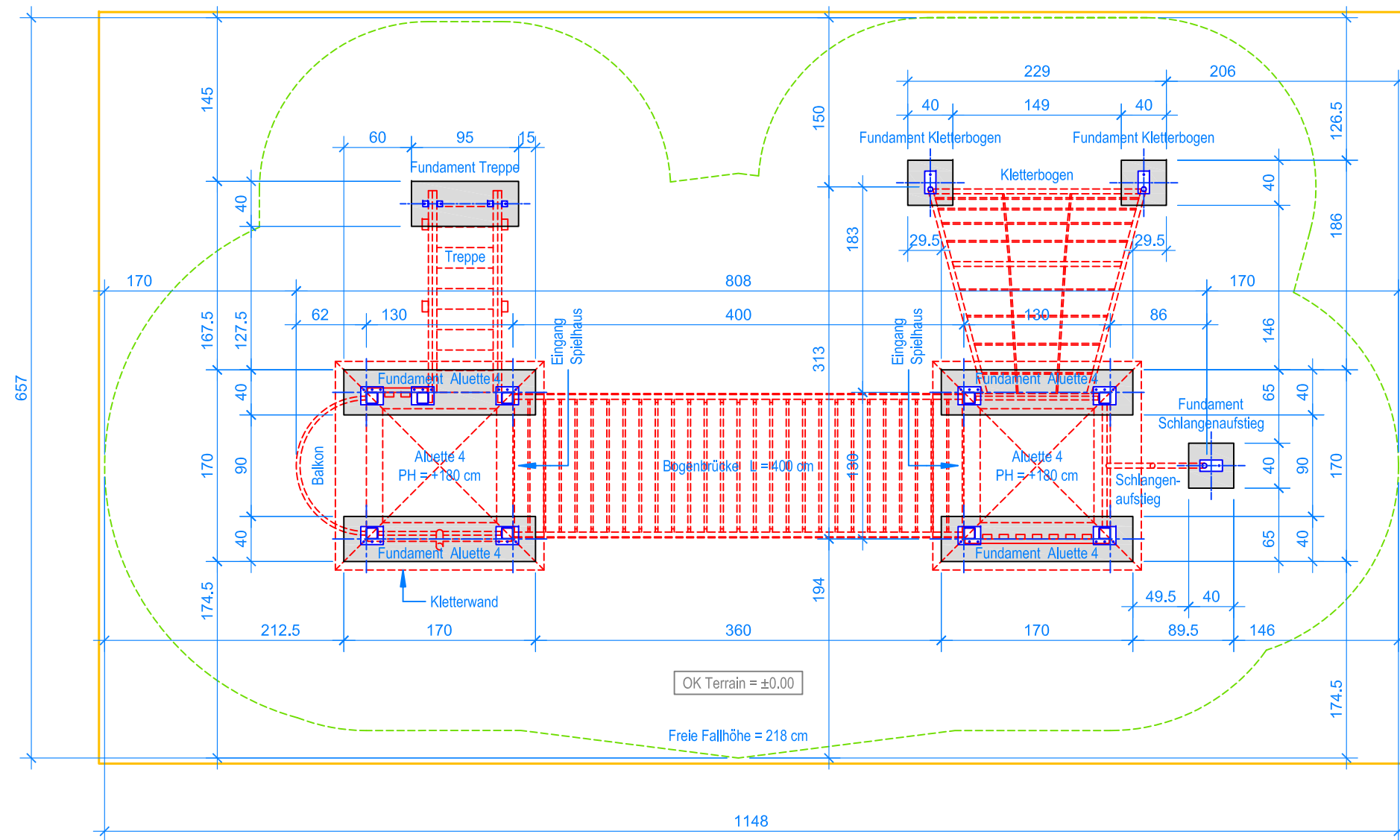
GRUNDRISS 1:50
