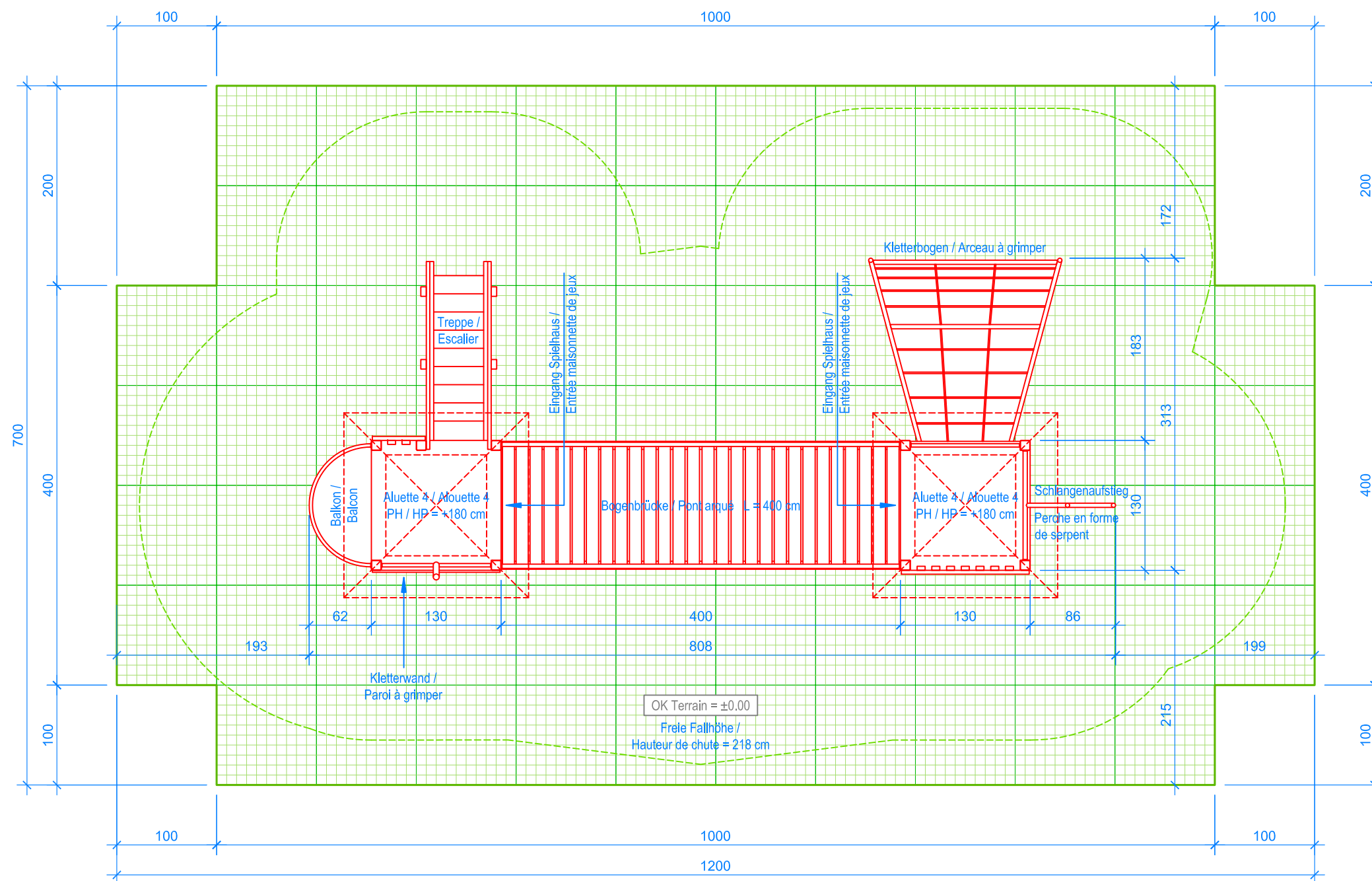
GRUNDRISS / PLAN 1:50
