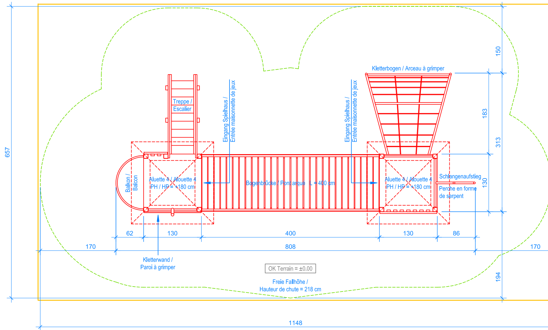
GRUNDRISS / PLAN 1:50
