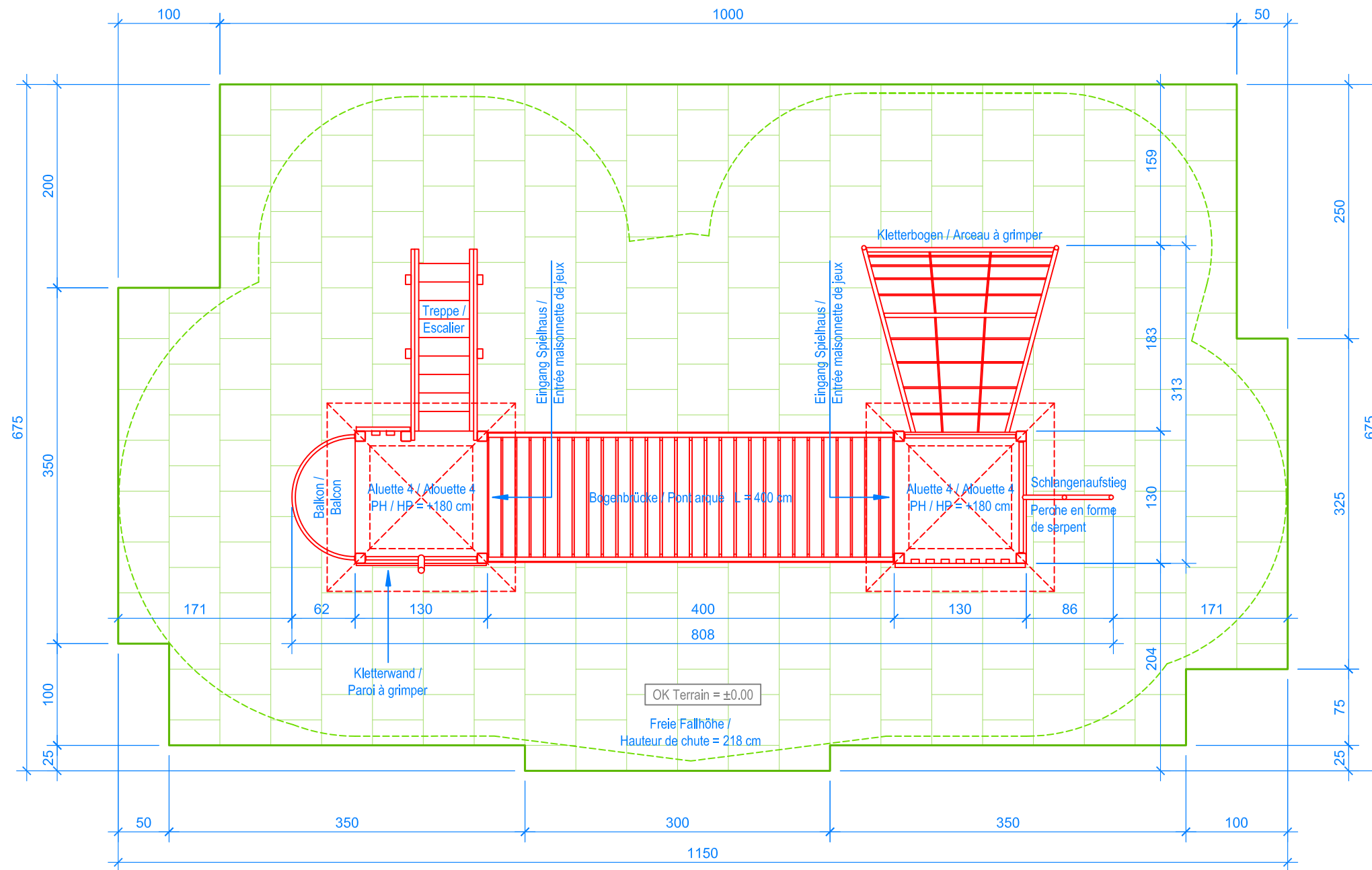
GRUNDRISS / PLAN 1:50
