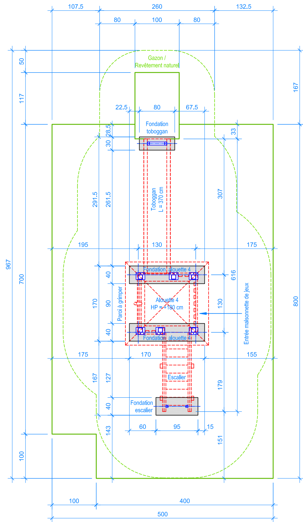
PLAN 1:50
