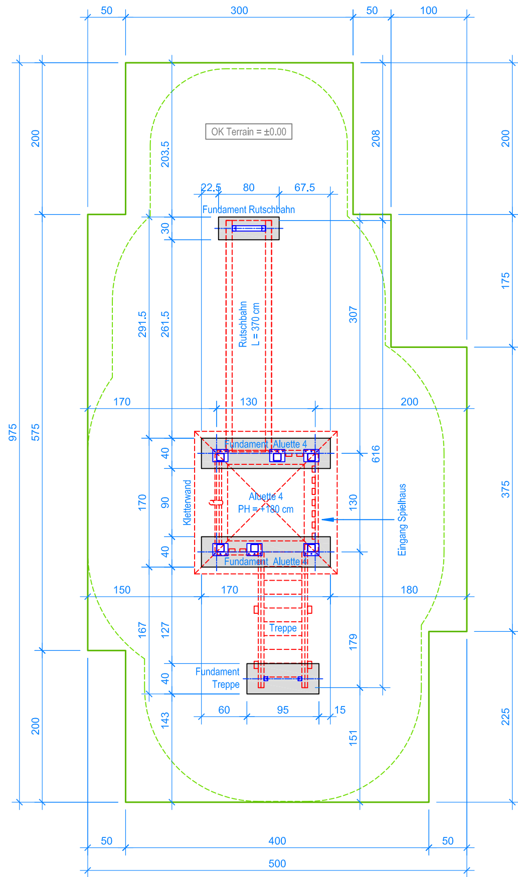
GRUNDRISS 1:50
