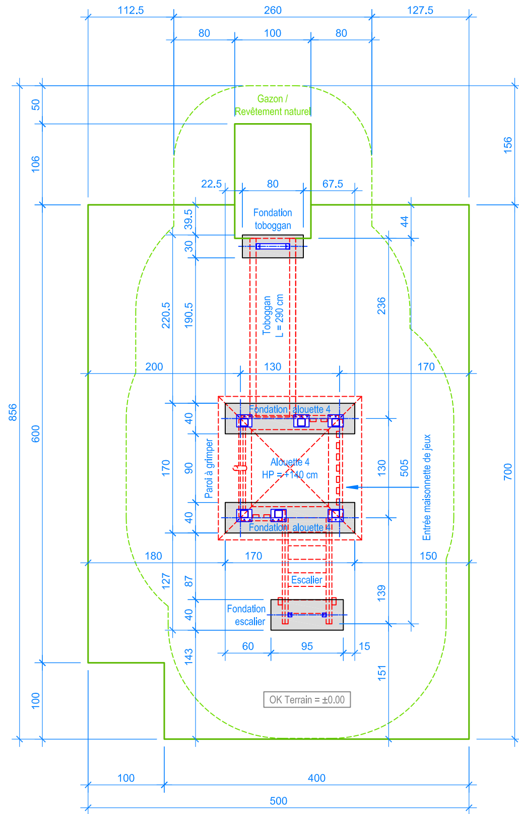
PLAN 1:50
