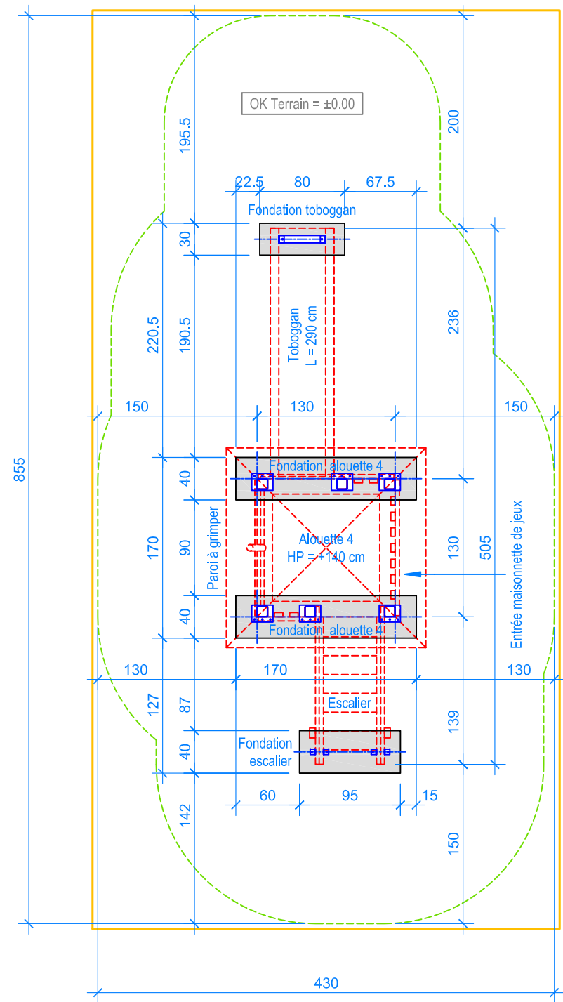
PLAN 1:50
