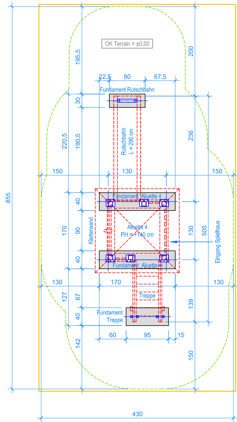
GRUNDRISS 1:50
