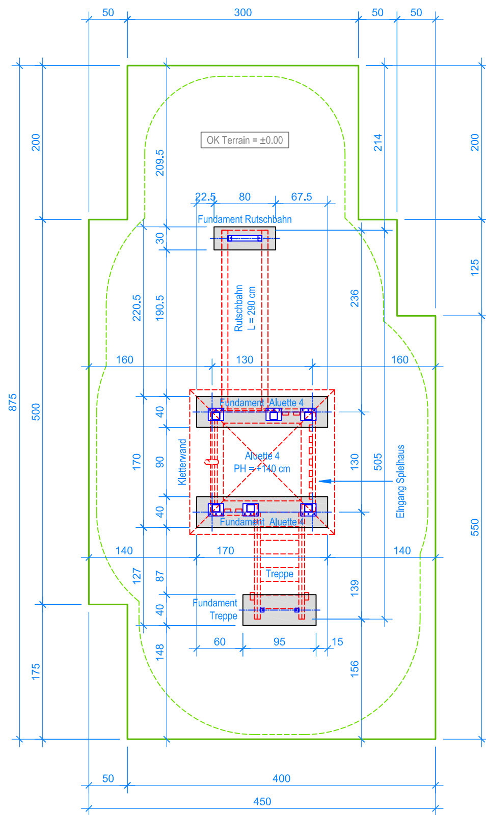
GRUNDRISS 1:50
